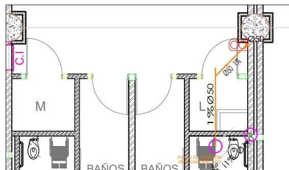
BAÑO CENTRAL
