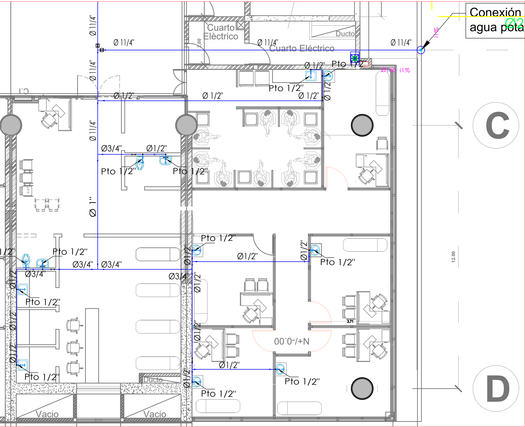
RED DE AGUA POTABLE
