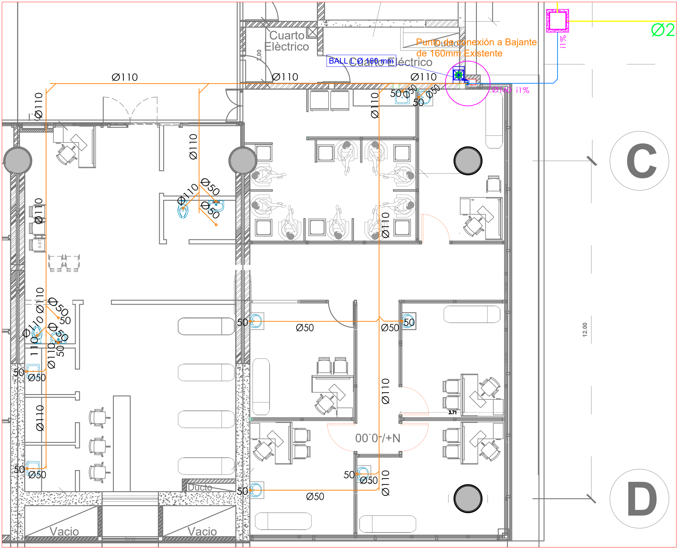
RED DE ALCANTARILLADO SANITARIO
